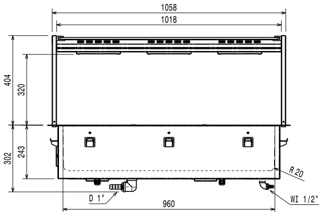
Front aanzicht
